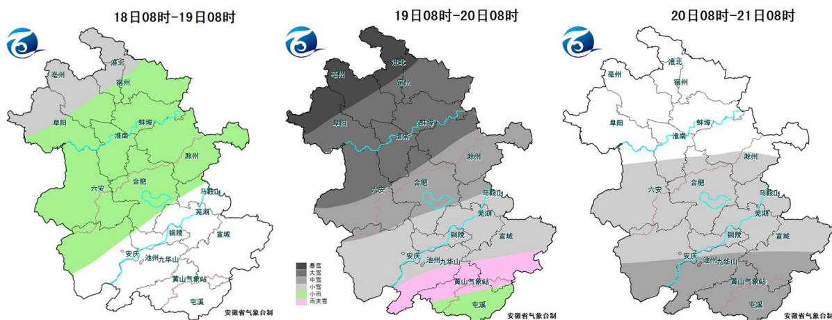
图 1 18-20 日全省雨雪落区图
