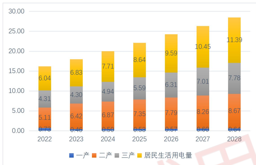
图 4-1 产值单耗法电量预测结果
