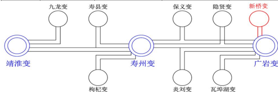
图 3-1 寿县 110kV 电网网架结构拓扑图
