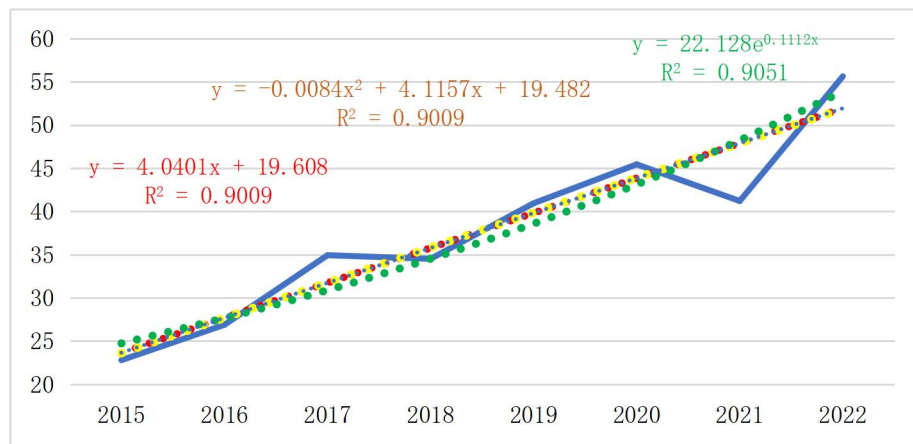
图 4-5 寿县历史负荷折线图
