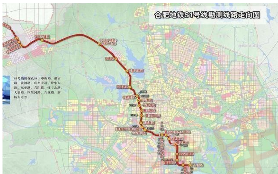
图 2- 5 合肥新桥机场 S1 线勘测线路走向图
