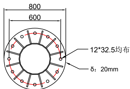
底部法兰示意图
