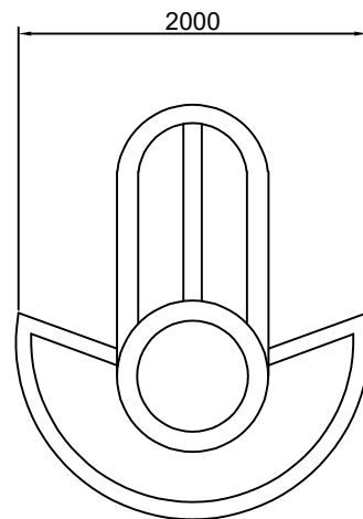
顶部6火灯盘示意图
